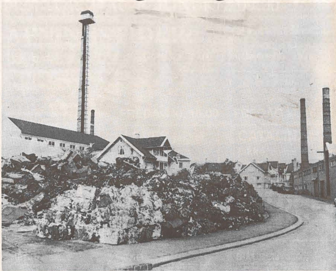
Hagltårnet med fabrikk under og smeltehuset på toppen - 60 meter over bakken. Legg merke til haugen av blikkavfall som skulle avtinnes.
