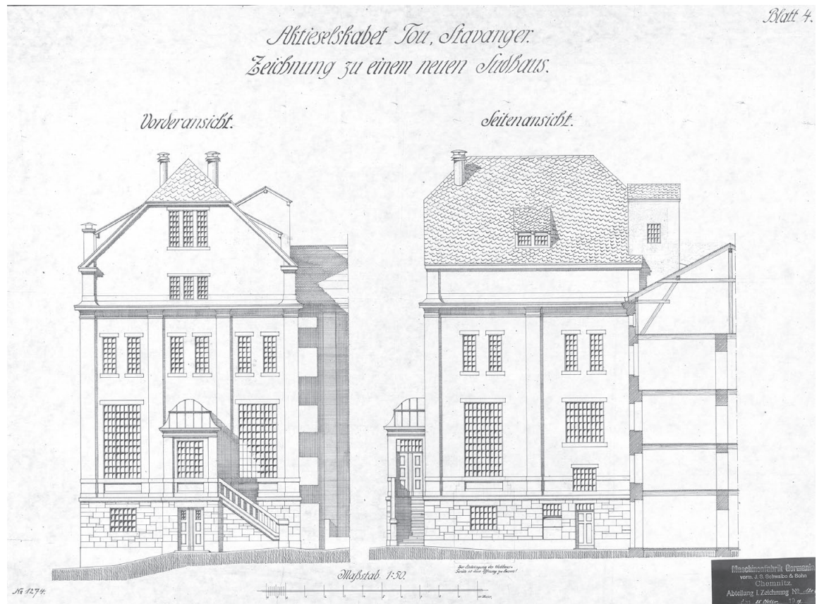
Arkitekttegninger av Tou Bryggeri. Nytt Tapperi. Fasade. Plansnitt. Datert 1923. Arkitekt Lars Storhaug. Byarkivet.
